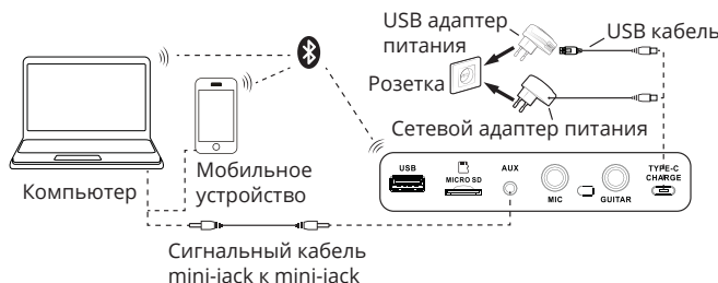
Рис.3. Схема подключения
